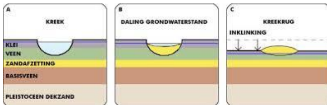
Afb 9 Proces van inklinking van de bodem
